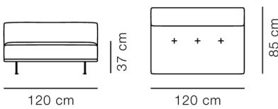
4502 Seat module 120x85 cm
