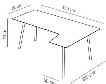
Return table 180x80
